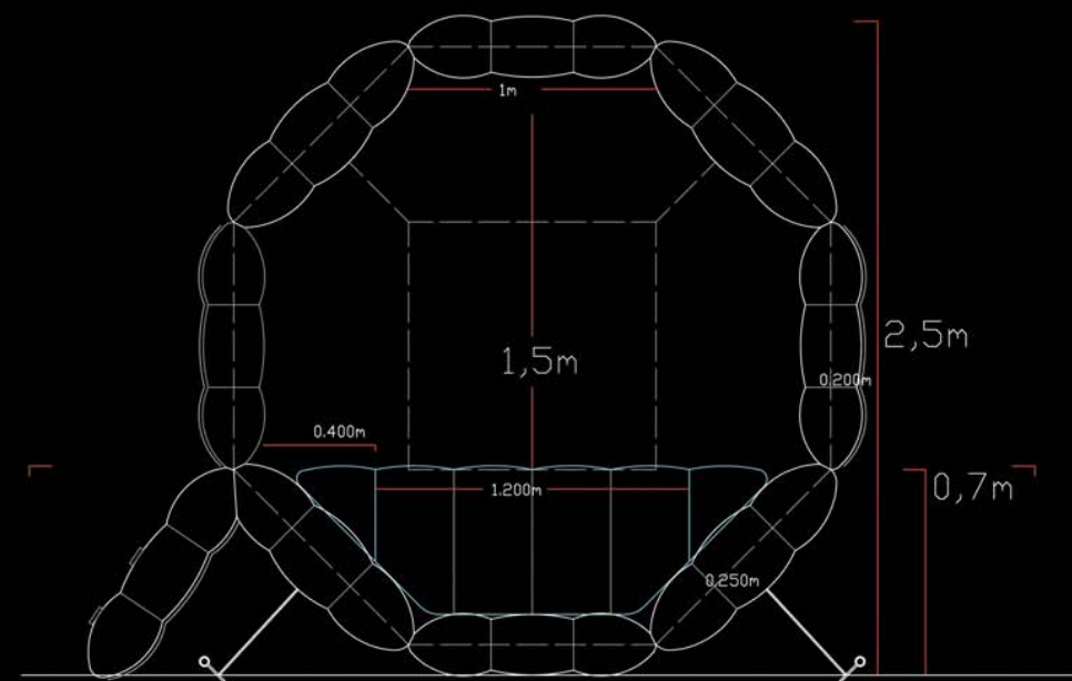
snitt 1:20
